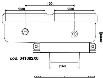
fig. 34- Accesoriu de pornire pentru conducte separate
