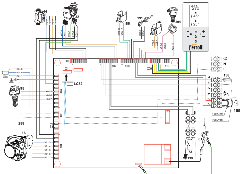
fig. 66- Schema electrică
