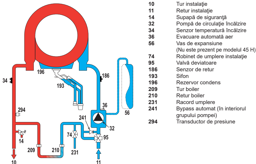
fig. 62- Circuitul hidraulic
